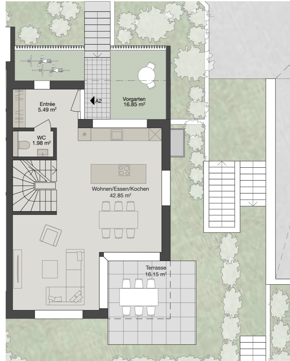
Erdgeschoss
