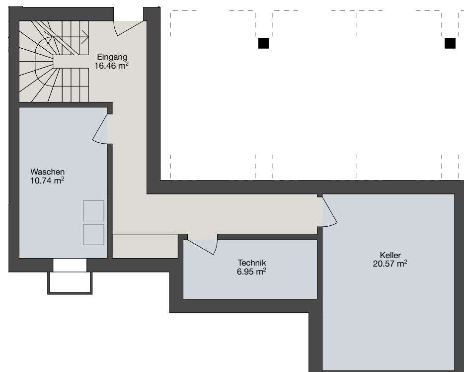
Untergeschoss
