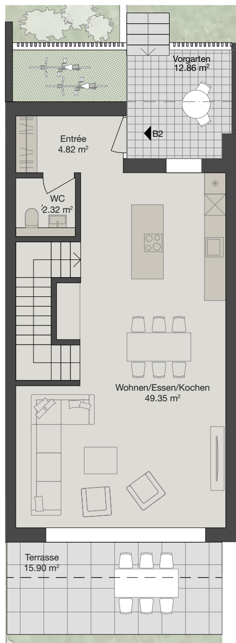
Erdgeschoss
